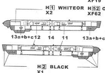
ALQ-119 ECM POD
