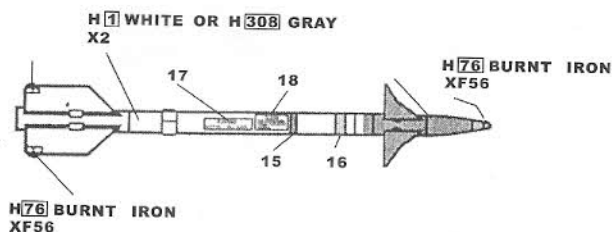
AIM-9L SIDEWINDER
